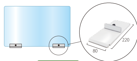
N20-94 メーカー直送 アクリルパーテーション W900×H600mm
