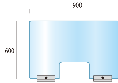
N20-95 メーカー直送 アクリルパーテーション 窓付 W900×H600mm 開口部 W300×H200mm
