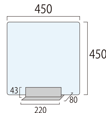
N20-96 メーカー直送 mini パーテーション透明 アクリル板：厚さ 1.5～2mm 角 R 付 ベース部：ステンレス
