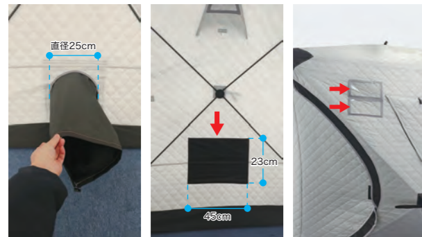
ダクト口(内側) ※排熱ホース用 ポケット(内側) ※ドレンホースの収納等に 差し込みポケット(外側) ※社名や注意書き等に 内寸:190x110mm
